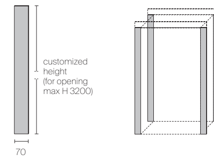
Back/front side filler
