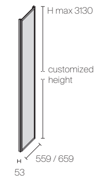
Back/front upper filler
