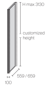
End panel (niche)
