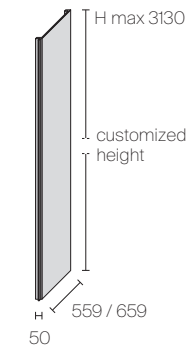
Back/front side filler
