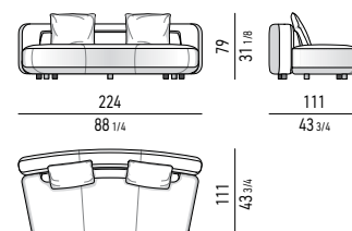
ELEMENTO CENTRALE CM 224 CENTRAL ELEMENT CM 224
